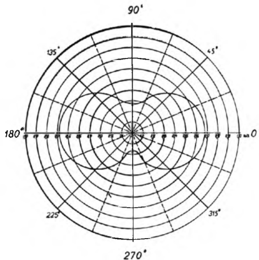
Fig. 9. Raam van 50 c M. Een punt in raamkring geard. Open dak-antenne, ontvanger geard.
