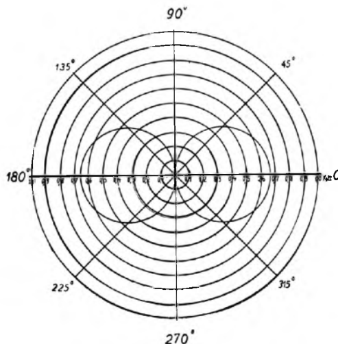
Fig. 14. Raam van 50 cm. Midden van raam geaard dak-antenne geaard ontvanger voorzien van in dit artikel omschreven geaard draad-scherm.
