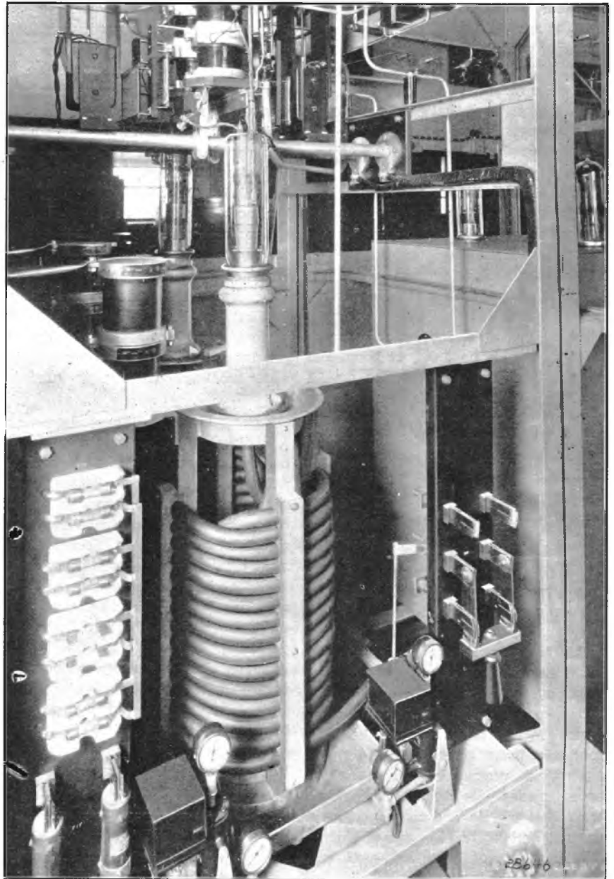
Een kijkje op de voorlaatste trap van een der krachtige kortegolf-zenders.
